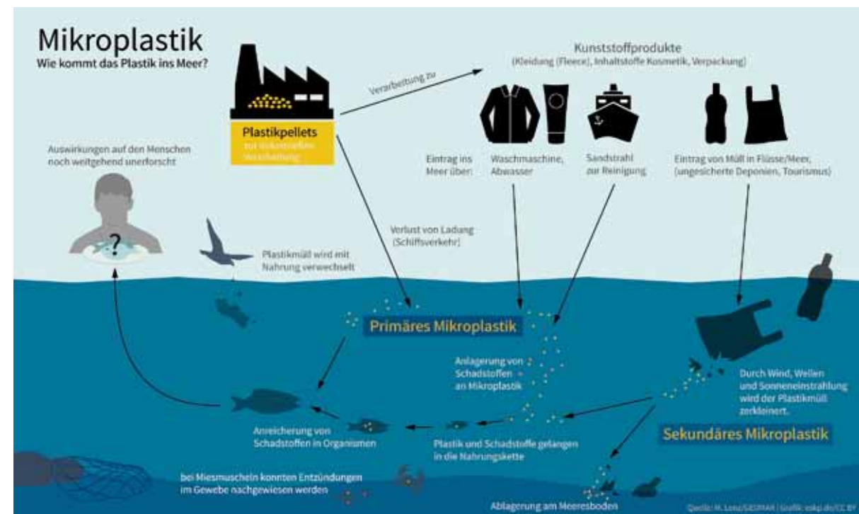
Wie kommt das Plastik ins Meer? Einträge von primären und sekundären Mikroplastik in die Ozeane.
