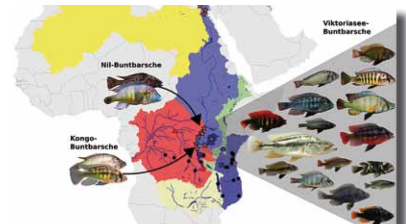
Die Flusssysteme rund um den Viktoriasee und die beiden ursprünglichen Vorfahren aus dem Nil- und dem Kongo-Einzugsgebiet sowie ein Teil der rund 700 aus ihnen hervorgegangenen Arten, 500 davon allein im Viktoriasee. Grafik: Eawag.
