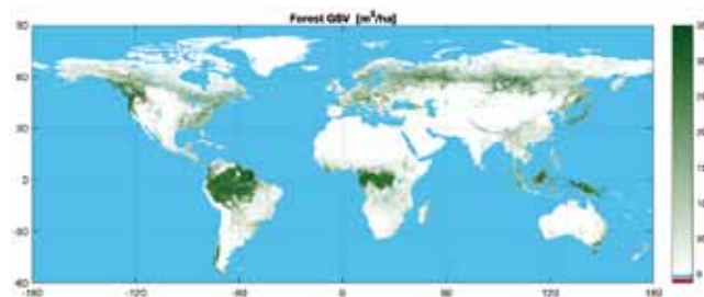
Eine globale Waldbiomasse-Karte hat die Europäische Weltraumbehörde jetzt veröffentlicht. Foto: ESA
